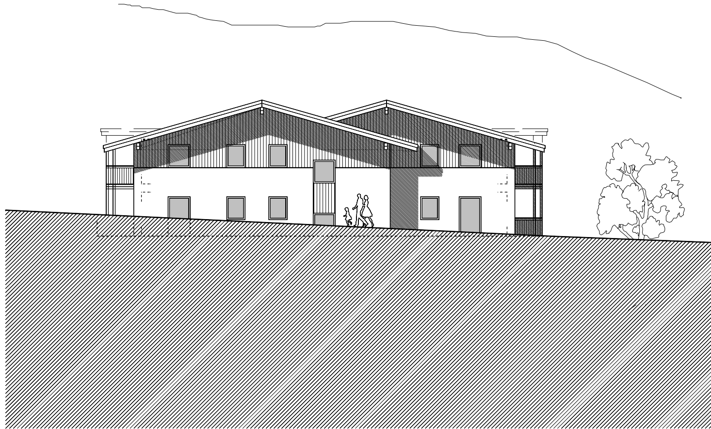
NORDANSICHT
