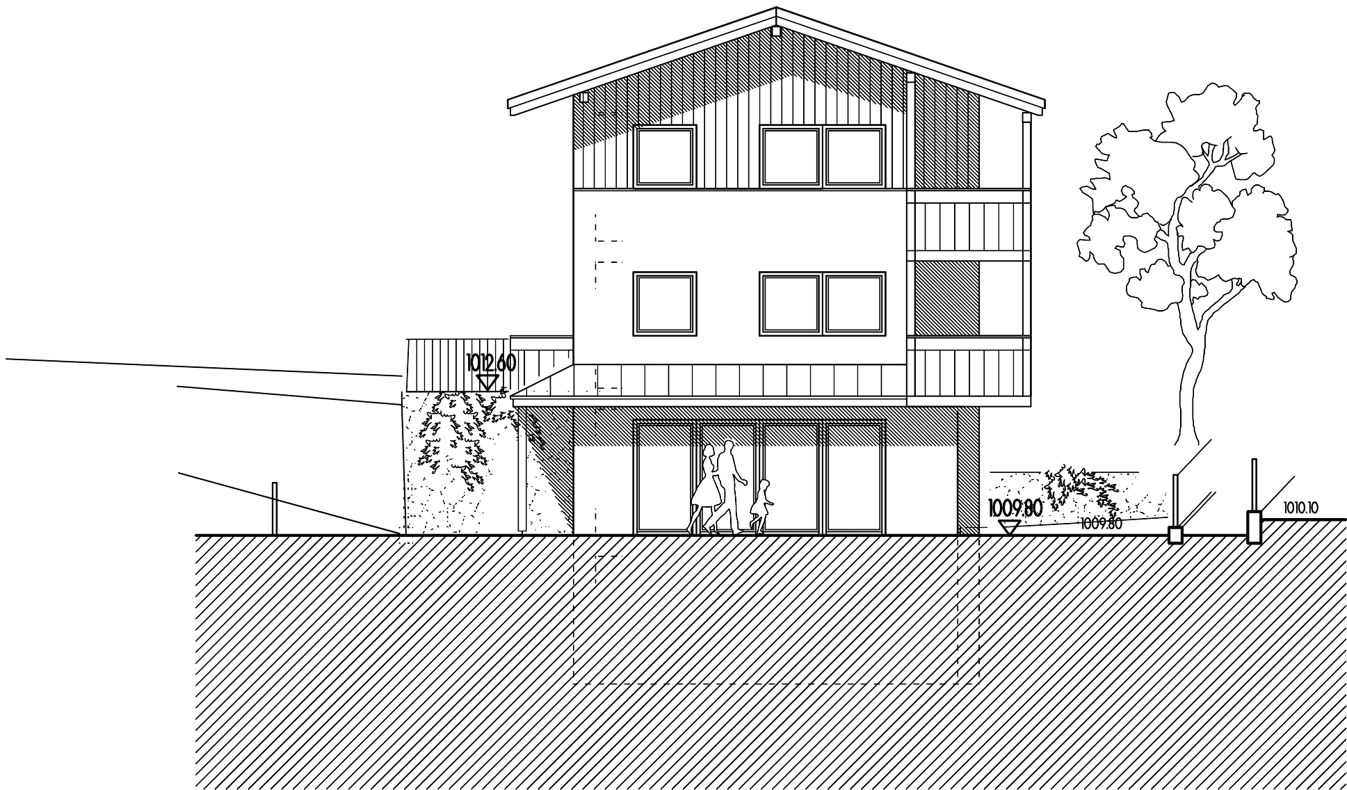
SUDWESTANSICHT
