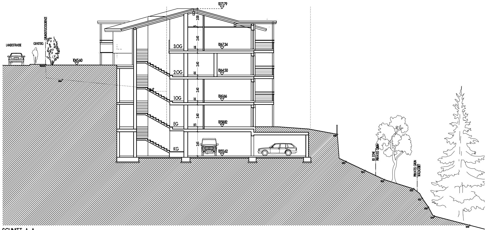
SCHNITT A-A
