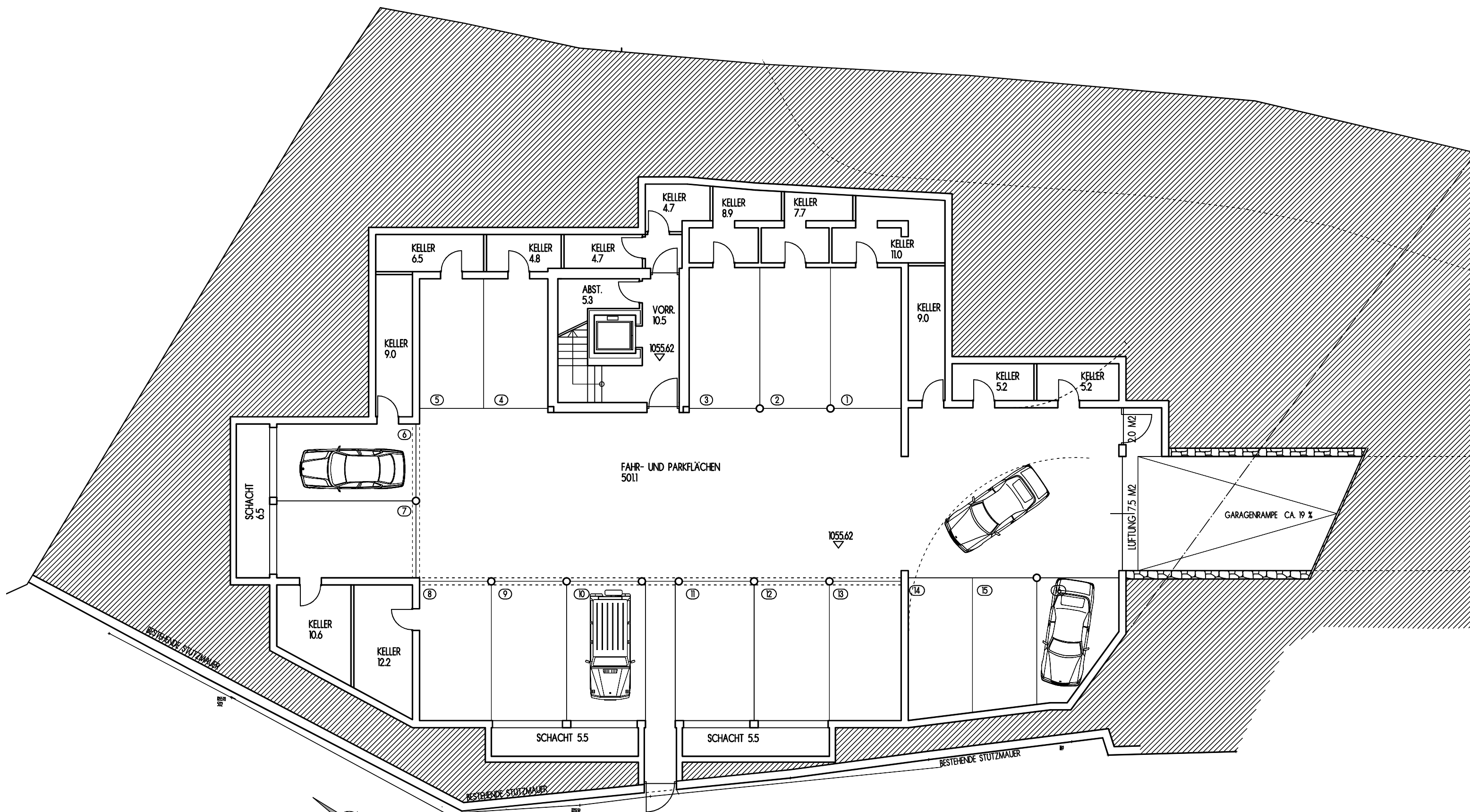
KELLER-GARAGENGESCHOSS
